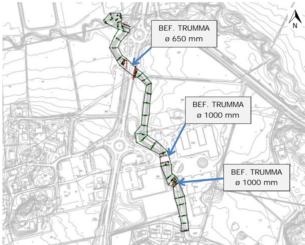
Figur 7. Visar inmätta tvärsnitt i grönt samt vägkanter och släntröner i rött. Tre trummor finns på den inmätta sträckan.
