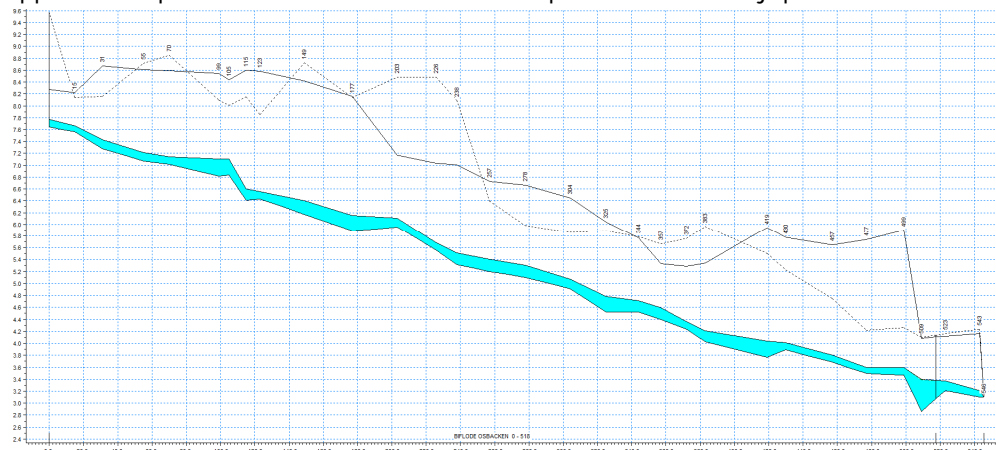
Figur 10. MQ för befintlig situation. Det blå visar vattennivån från botten till ytan. Linjerna med siffror visar slänkrönet för respektive tvärsnitt.
