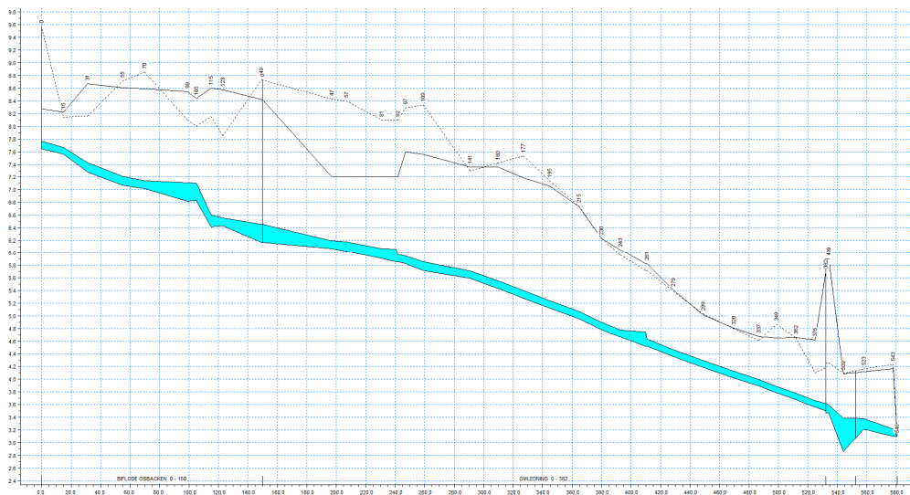
Figur 11. MQ för situation med omledning av bäck. Det blå visar vattennivån från botten till ytan. Linjerna med siffror visar slänkrönet för respektive tvärsnitt.
